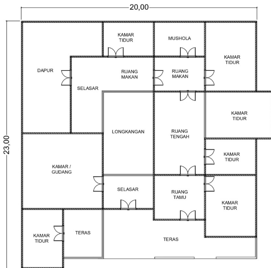
DENAH BANGUNAN LOJI MANGGORAN
